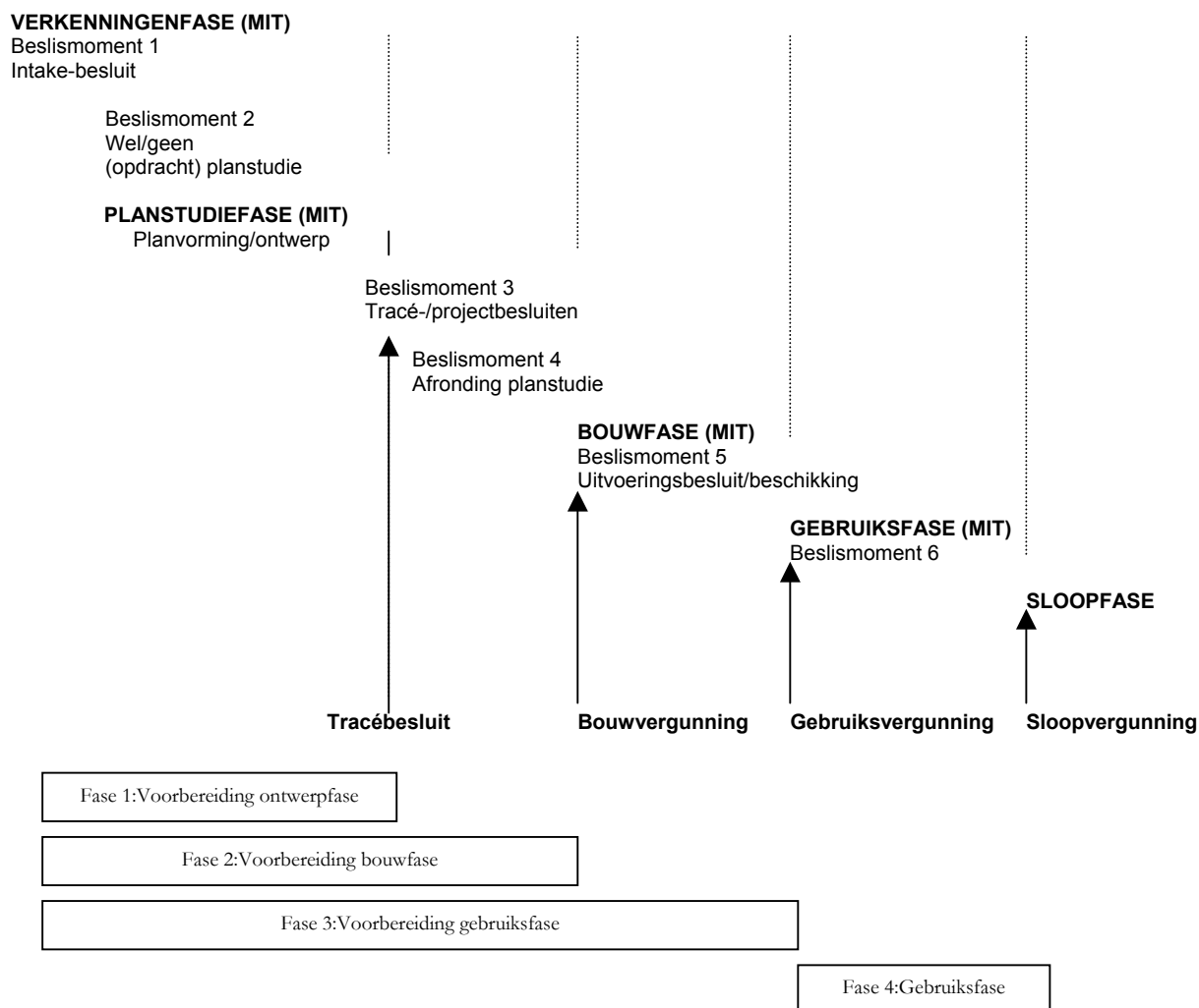
Figuur 1.1 - Fasering en beslismomenten tunnelveiligheid
