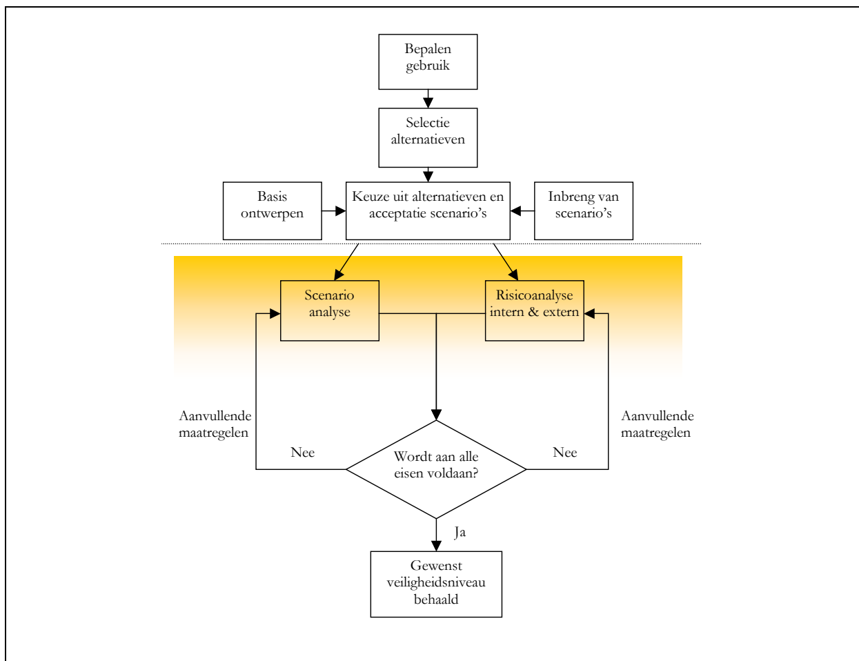
Figuur 5.1: Methodiek voor een veilige tunnel
